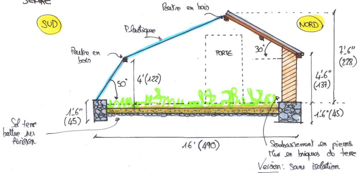
COUPE A'A DE PRINCIPALE
